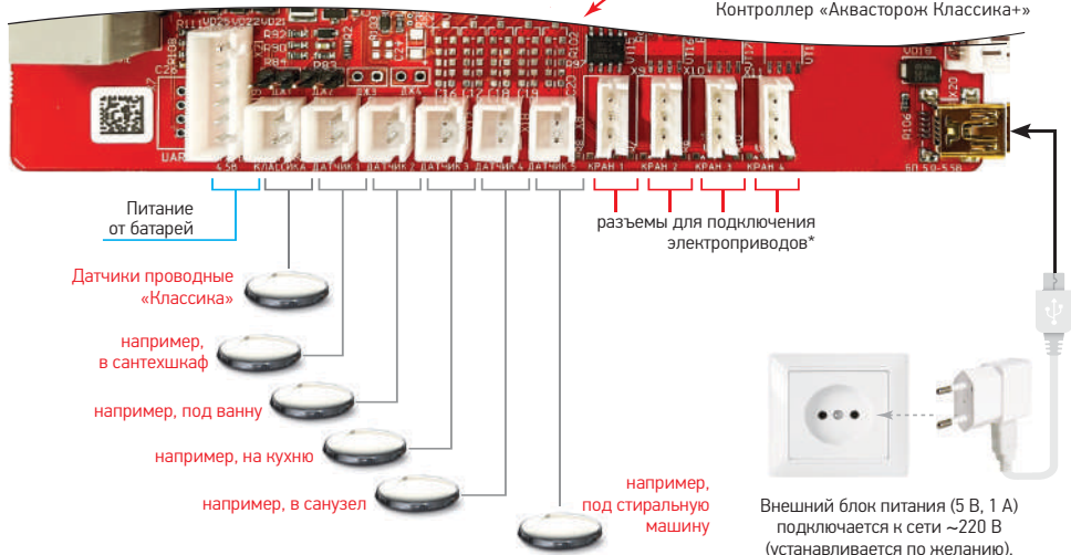
Контроллер «Аквасторож Классика+»
