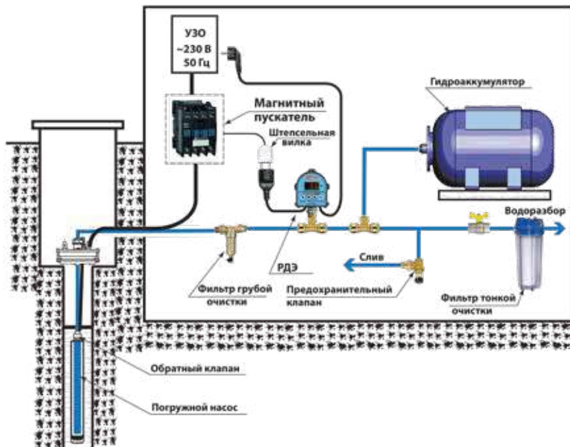
Пример 4. Подключение РДЭ для управления однофазным насосом мощностью P1 более 1,5 кВт, или трехфазным погружным насосом.
