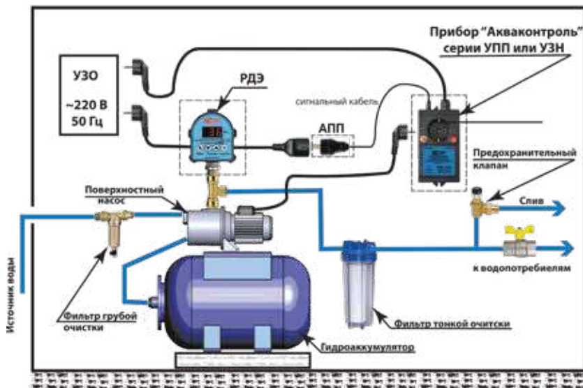
Пример 3. Подключение РДЭ к УПП или УЗН “Extra Акваконтроль” через адаптер АПП.
