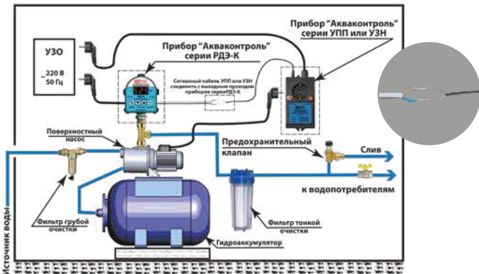
Пример 6. Подключение РДЭ-К к УПП или УЗН "Extra Акваконтроль" без использования адаптера АПП.
