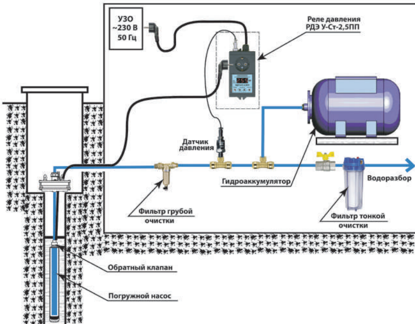
Пример подключения РДЭ У-Ст-2,5ПП “Акваконтроль” с погружным насосом (плавный пуск, P1max=2,5кВт).
