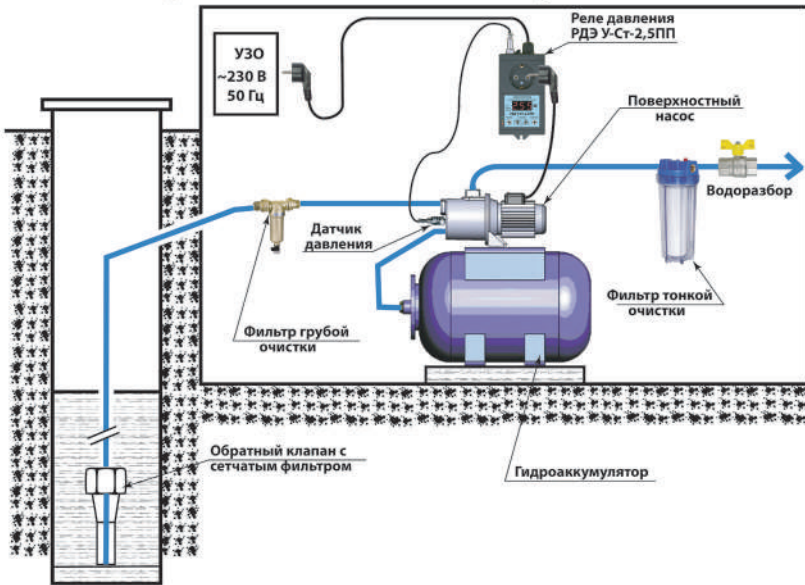
Пример подключения РДЭ У-Ст-2,5ПП “Акваконтроль” с поверхностным насосом (плавный пуск, P1max=2,5кВт).
