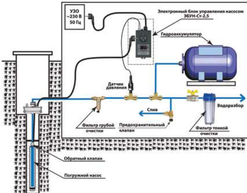
Пример 4. Подключение приборов серии ЭБУН-Ст к погружному насосу.
