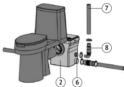
Рисунок 2 – Устройство КНС
