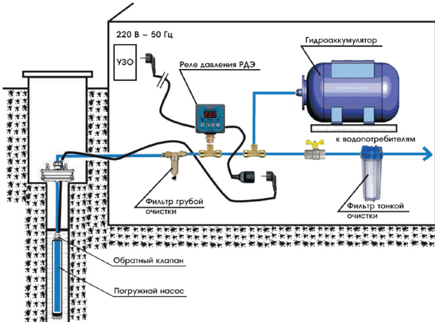
Схема 2. Подключение реле давления РДЭ "Акваконтроль" с погружным насосом
