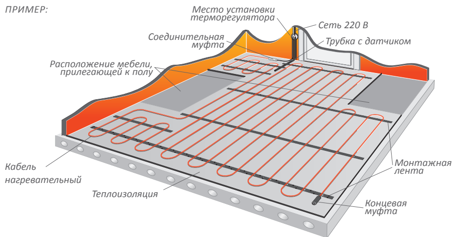
Схема раскладки двужильного нагревательного кабеля
