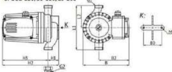
UPC 32-120, 25-160, 25-200
