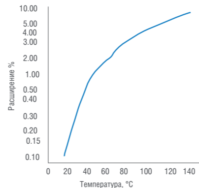
РАСШИРЕНИЕ ВОДЫ ИЗ-ЗА РАЗНИЦЫ ТЕМПЕРАТУР
