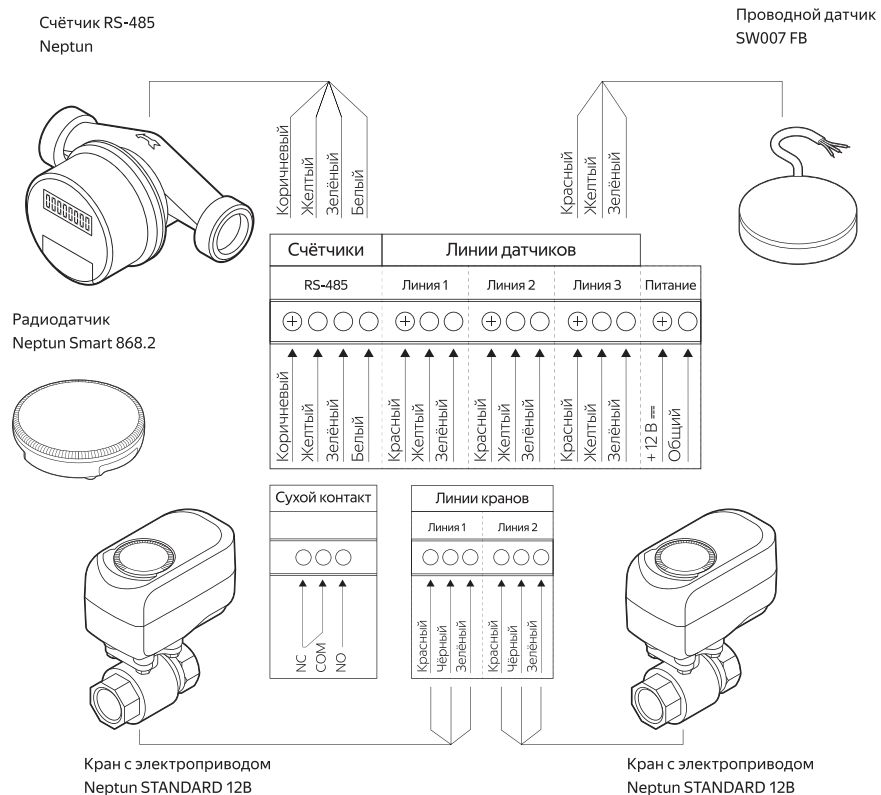
Рисунок 6. Схема подключения
