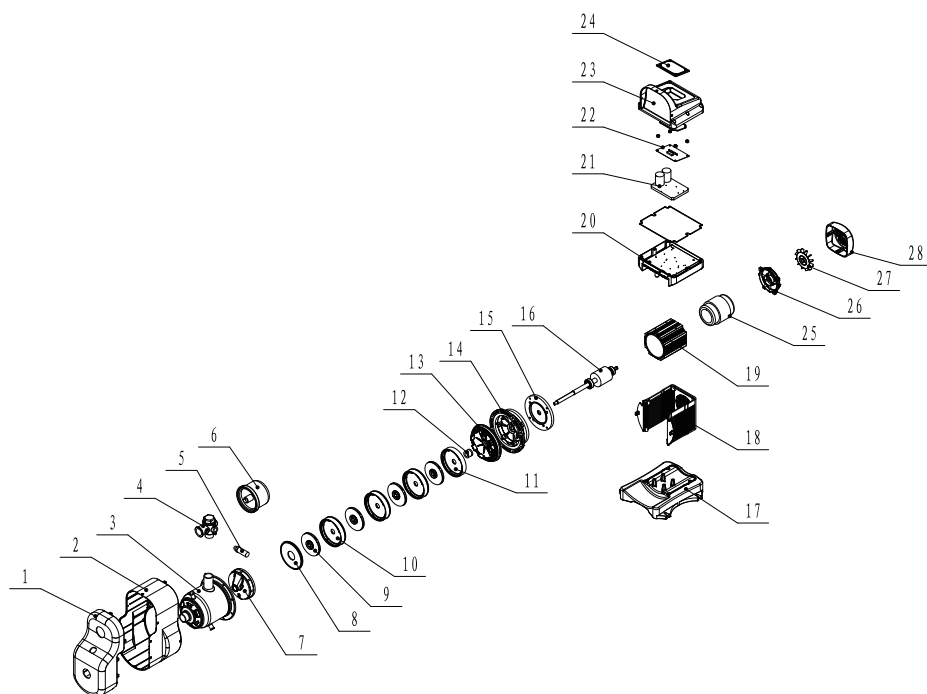
Рисунок 3 – Конструкция станции
