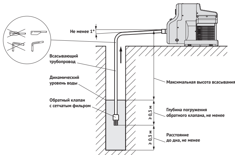
Рисунок 4 – Гидравлическое подключение
