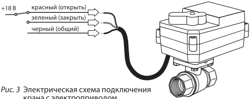
Рис. 3 Электрическая схема подключения крана с электроприводом серии Neptun Bugatti Pro 18 B
