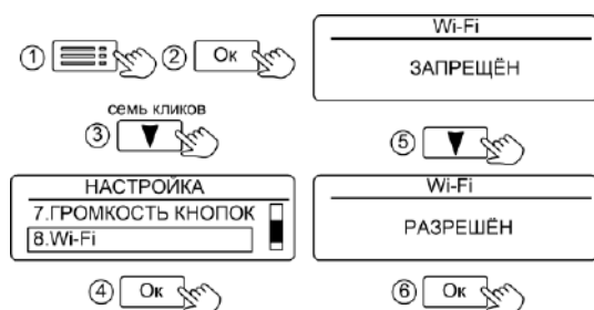
Рисунок 22. Включение Wi-Fi
