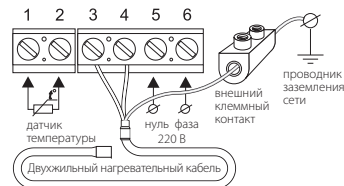
Схема подключения к 3-х проводной электрической сети
