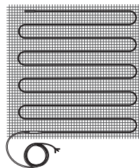
Нагревательный мат ProfiMat
