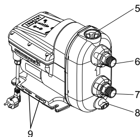
Рис. 22 Установка SCALA2
