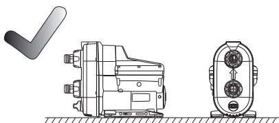
Рис. 4 Установка на горизонтальном основании
