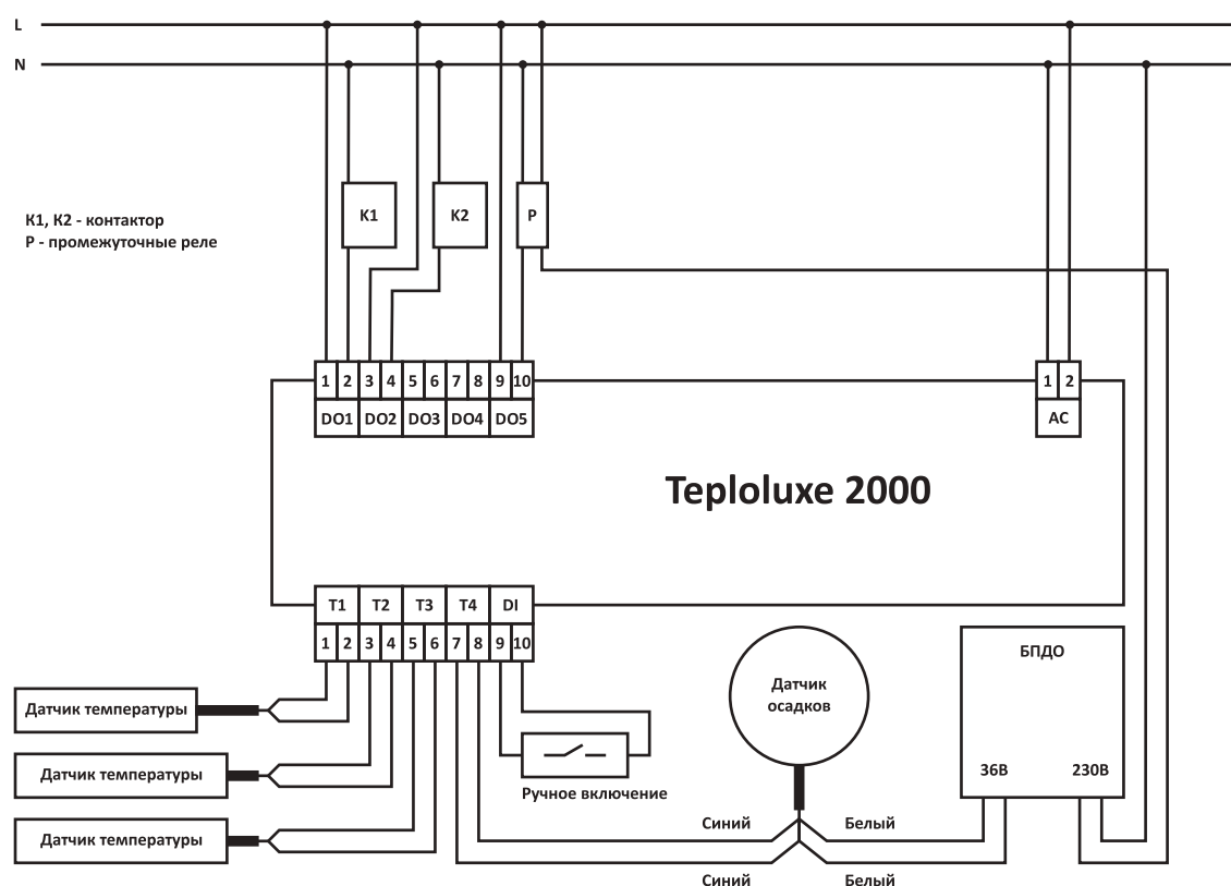
Рис. 3.3.1 Принципиальная схема подключения в режиме «Двор»
