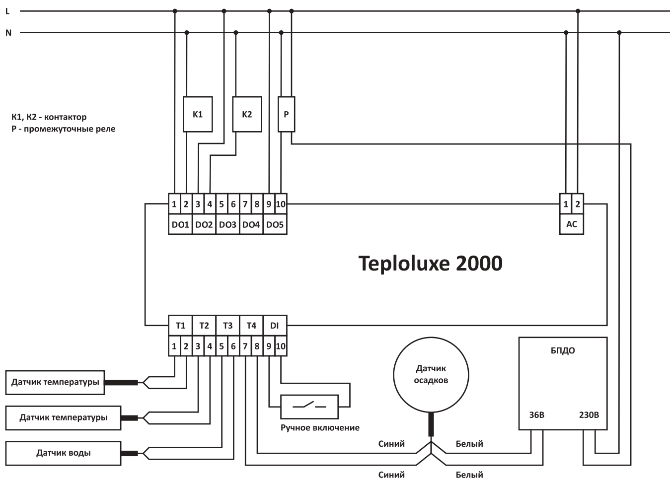
Рис. 3.2.1. Принципиальная схема подключения в режиме «Кровля/Двор»
