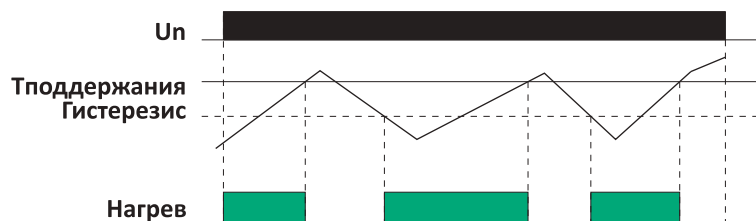
Рис. 3.3.3. Принцип работы гистерезиса
