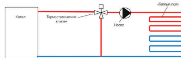
Рис.2 Пример применения смесительного термостатического клапана
