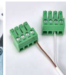
Фото 10. Подключение провода датчика к ответной части разъема электропривода
