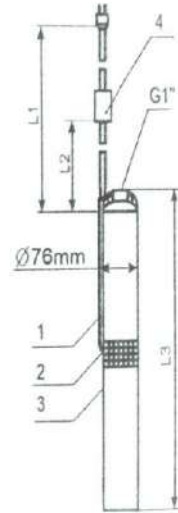
Рис. 1. Габаритные и присоединительные размеры
